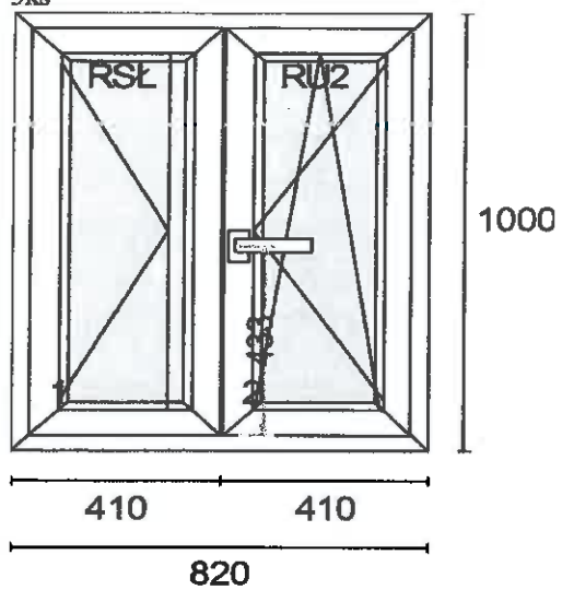
Prvek č. 7 – dvě křídla s pohyblivým sloupkem napravo 4 ks
